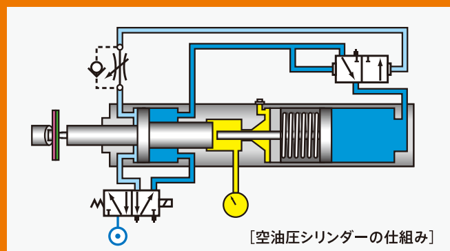
【空油圧シリンダーの仕組み】
