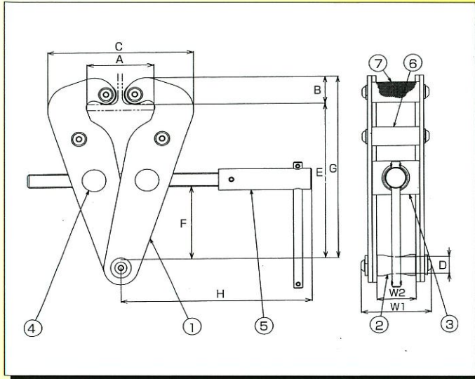
寸法図
